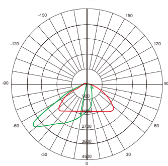
AST-S-G20-240WXYDA1
